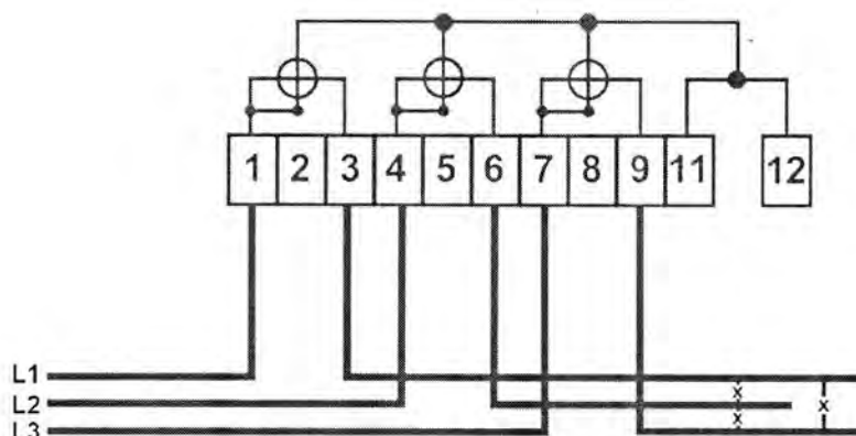
Рисунок 14. Схема включення в 3-х провідну мережу лічильників безпосереднього підключення запрограмованих на включення у 4-х провідну мережу з 3-ма вимірювальними елементами
