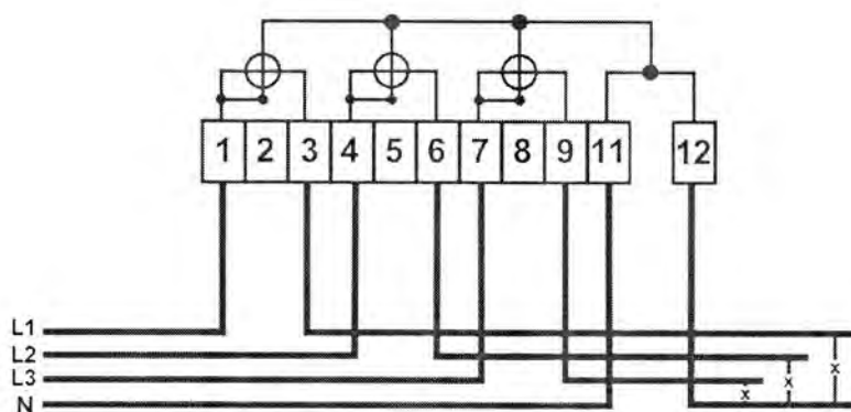
Рисунок 13. Схема включення в 4-х провідну мережу лічильників безпосереднього підключення запрограмованих на включення у 4-х провідну мережу з 3-ма вимірювальними елементами
