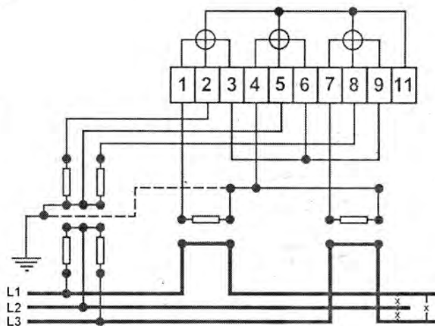
Рисунок 12. Схема включення в 3-х провідну мережу лічильників трансформаторного підключення запрограмованих на включення у 4-х провідну мережу з 3-ма вимірювальними елементами
