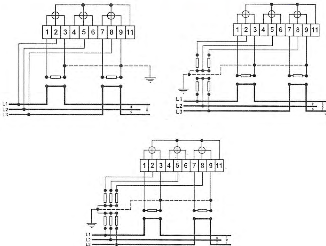
Рисунок 11. Схема включення в 3-х провідну мережу лічильників трансформаторного підключення запрограмованих на включення у 3-х провідну мережу з 2-ма вимірювальними елементами
